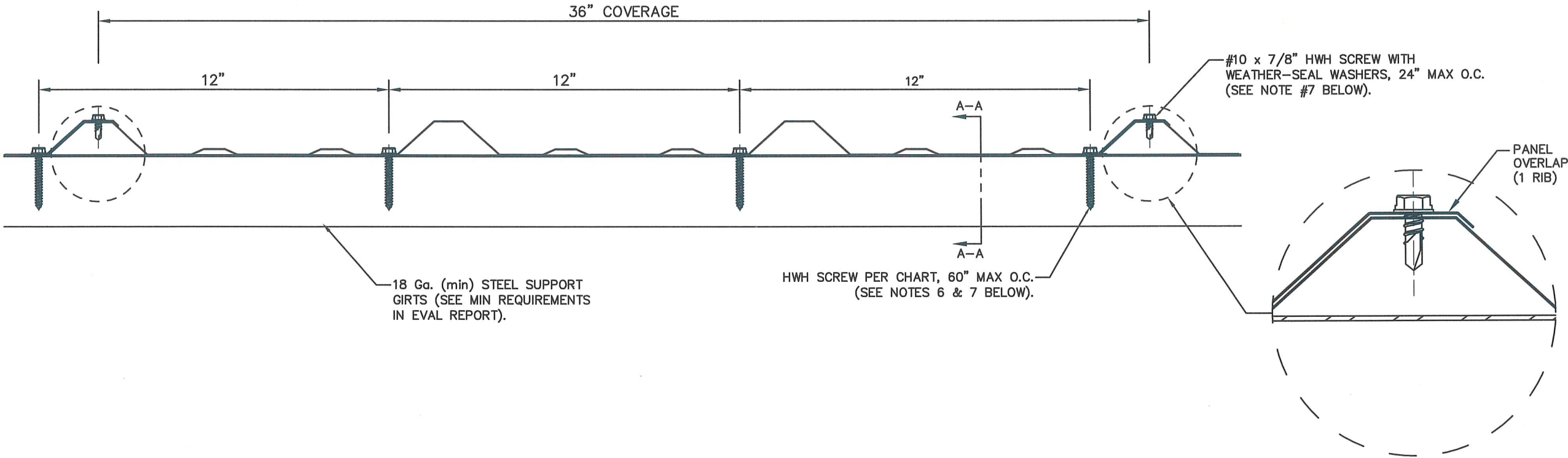
SECTION A-A
